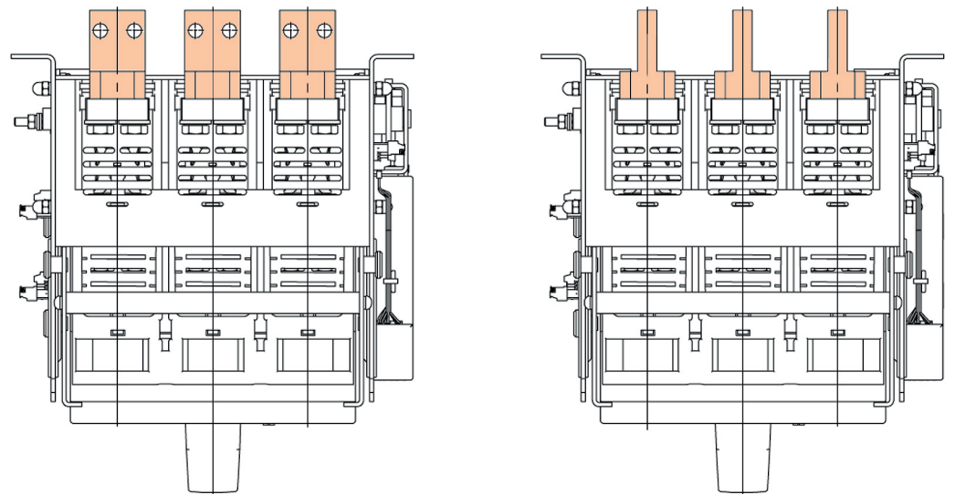
б) выдвижное исполнение выключателя
