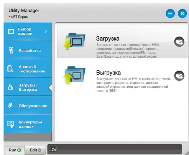
Рисунок 4.25 – Окно «Загрузка/Выгрузка» ПО Utility Manager
