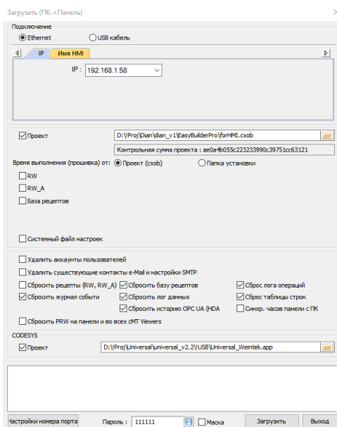
Рисунок 4.12 – Окно «Загрузить (ПК-&gt;Панель)» ПО Utility Manager
