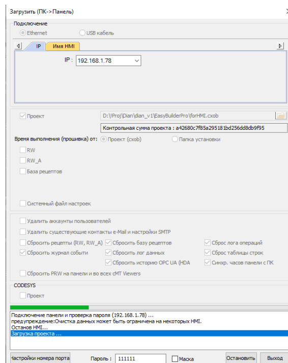
Рисунок 4.28 – Процесс загрузки прикладного ПО
