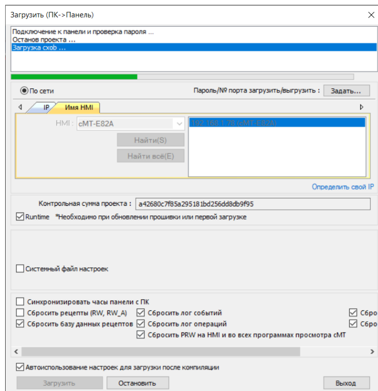
Рисунок 4.23 – Процесс загрузки прикладного ПО в панель оператора
