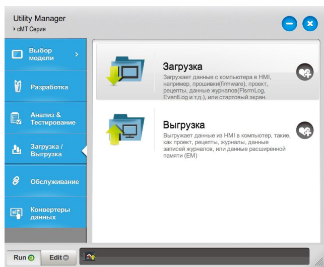
Рисунок 4.11 – Окно «Загрузка/Выгрузка» ПО Utility Manager
