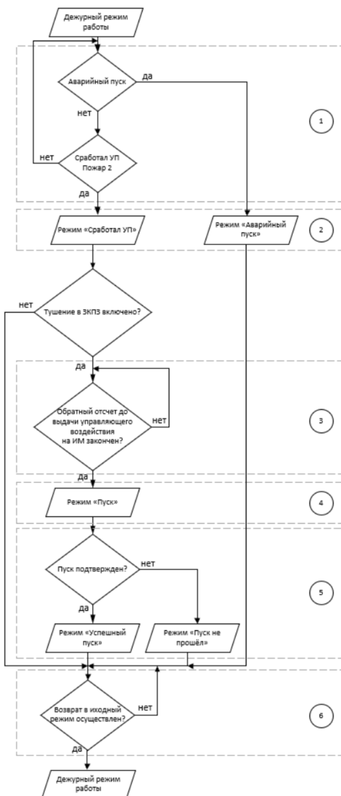
Рисунок 4.1 – Алгоритм фиксации режимов «Аварийный пуск», «Пуск (выдача сигнала на ИМ противопожарной защиты)», «Сработал УП» в дежурном режиме работы ЗКПЗ
