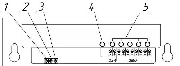
Схема подключения ББП-50 М v5
