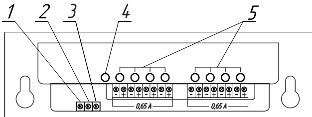
Схема подключения ББП-50 М v8
