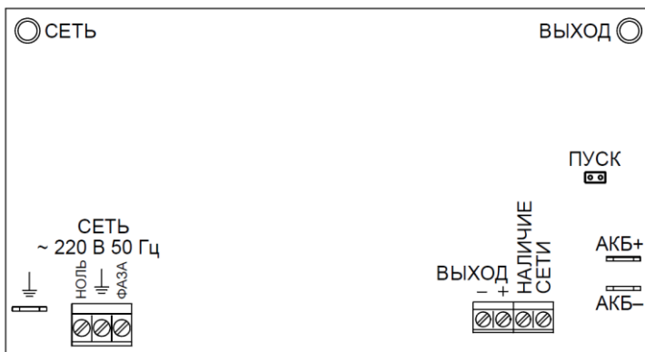
Рисунок 2 - Общий вид платы
