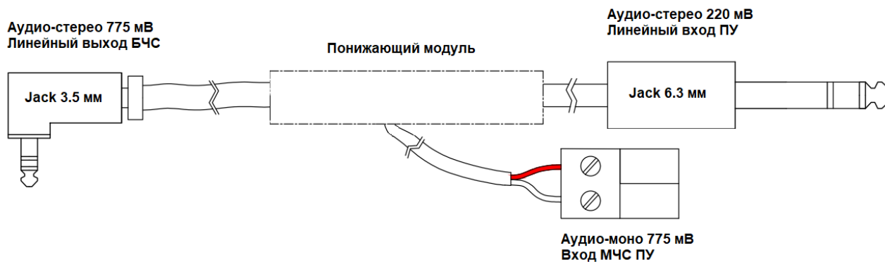
Рисунок 5 - Аудио кабель подключение (в комплекте)
