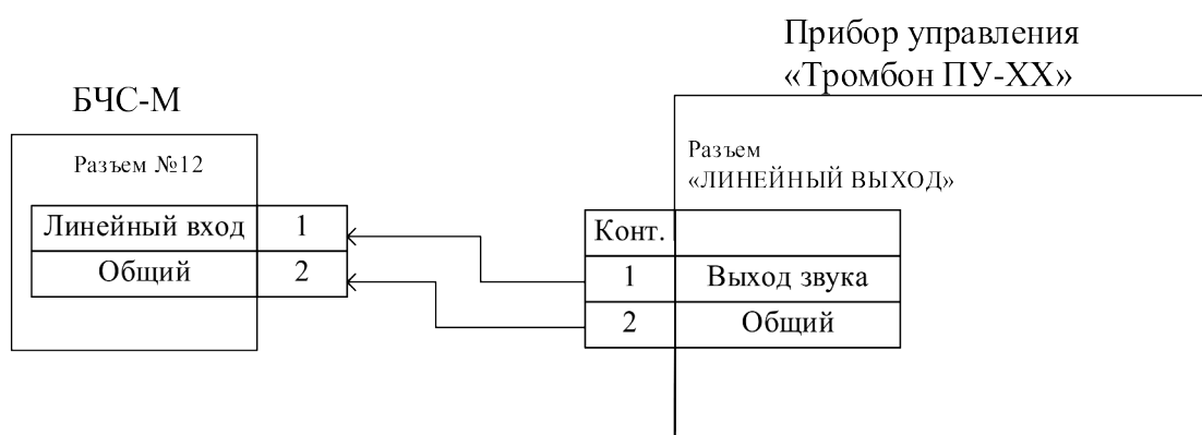
Рисунок 6 - Схема подключения аудио кабеля для связи «Тромбон БЧС-М» с прибором управления «Тромбон ПУ-ХХ»
