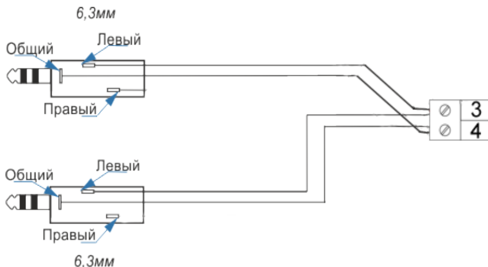
Рисунок 7 - Схема разводки аудио кабеля для связи «Тромбон БЧС-М» с прибором управления «Тромбон ПУ-ХХ»
