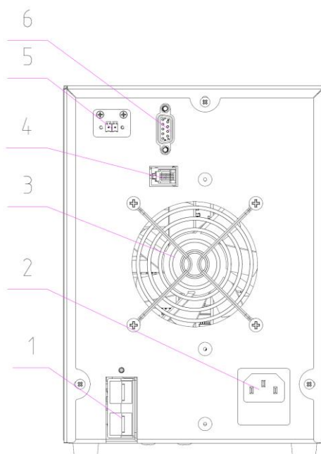
Рисунок 1.2 – Зарядное устройство Штиль ВСТ-36. Вид с фронтальной стороны
