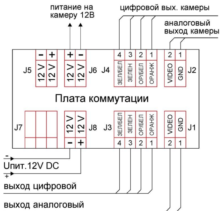
Рисунок 4в – Подключение исполнений 01
