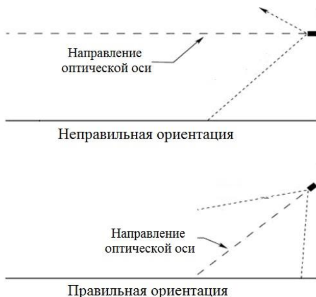
Рисунок 5 – Установка термокожуха с ИК-прожектором по отношению к горизонту
