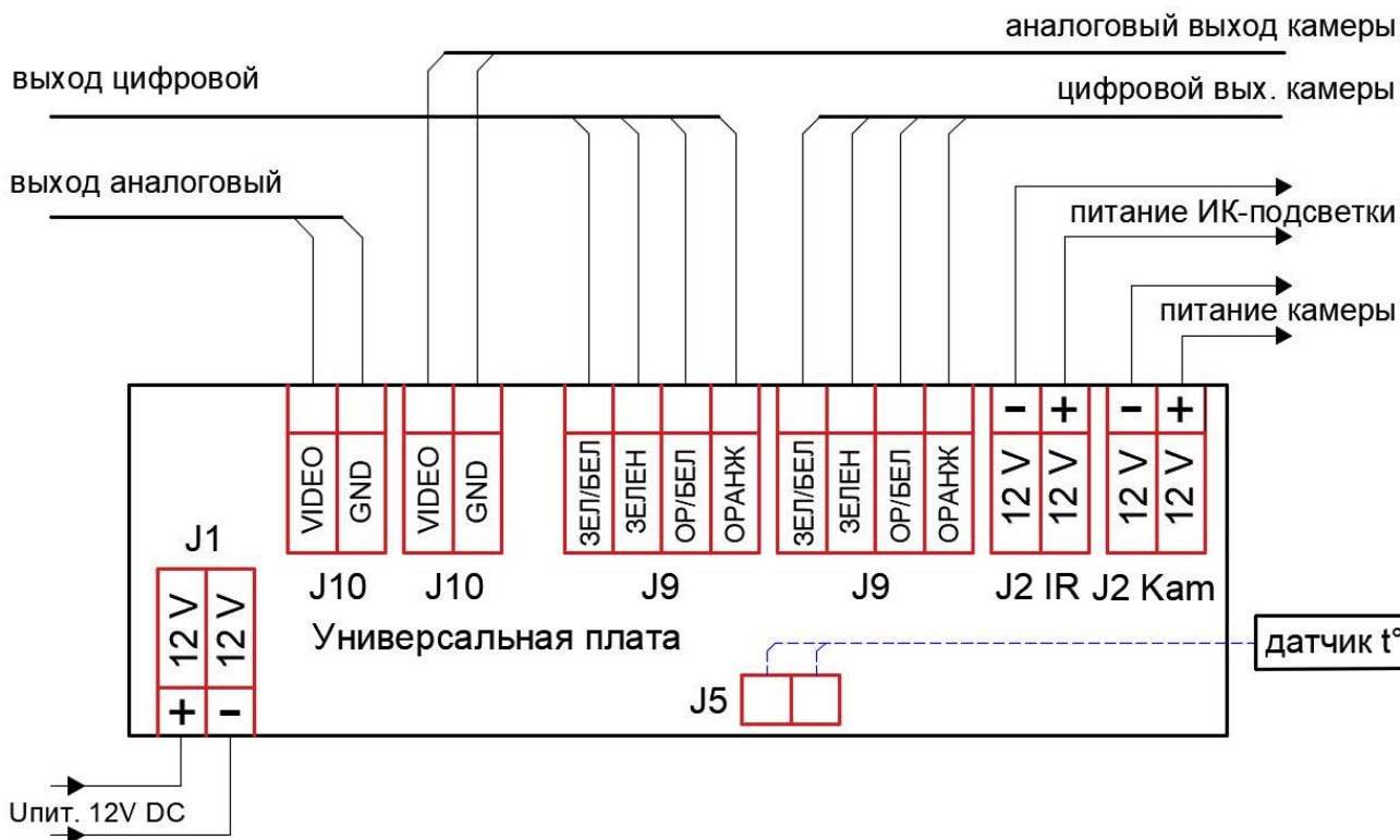
Рисунок 6б – Схема подключения термокожуха с напряжением питания 12 В от инжектора
