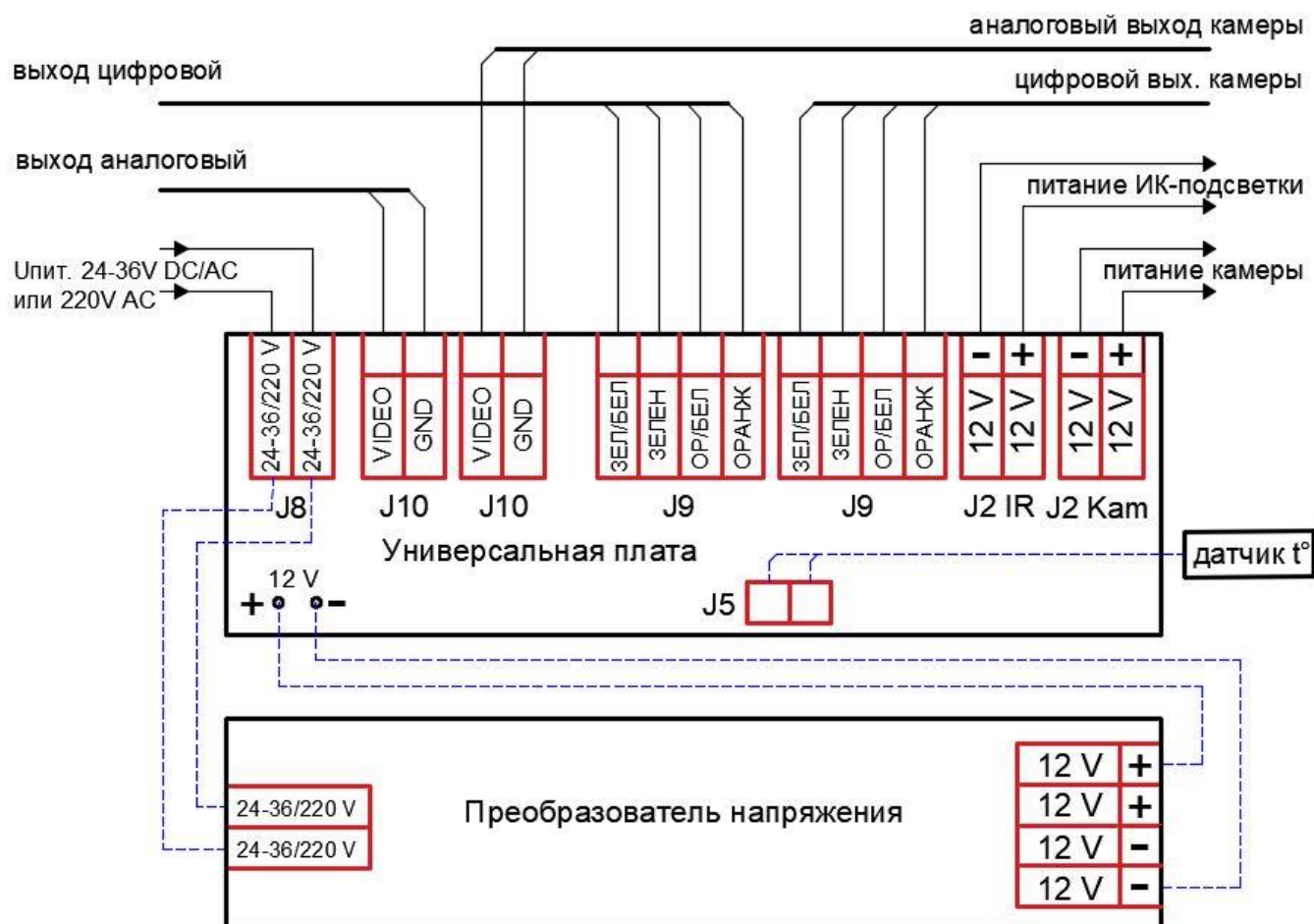
Рисунок 6а – Схема подключения термокожуха с напряжением питания 24-36 В и 220 В.
