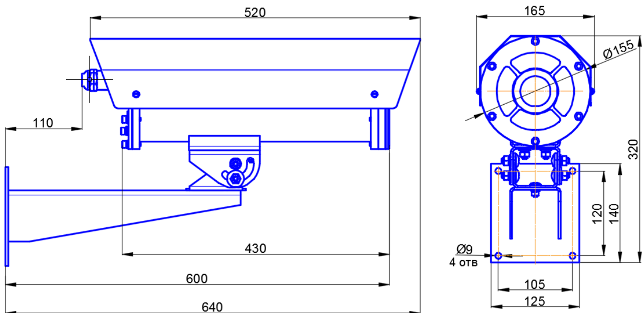
Рисунок 1 – Габаритные размеры термокожуха с ИК-прожектором
