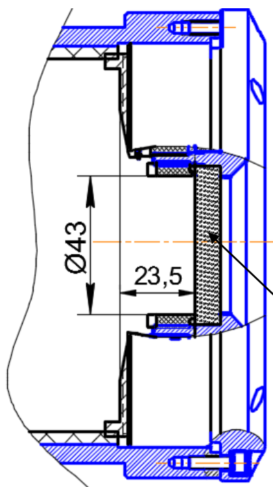
Рисунок 2 – Внутреннее пространство смотрового окна.
