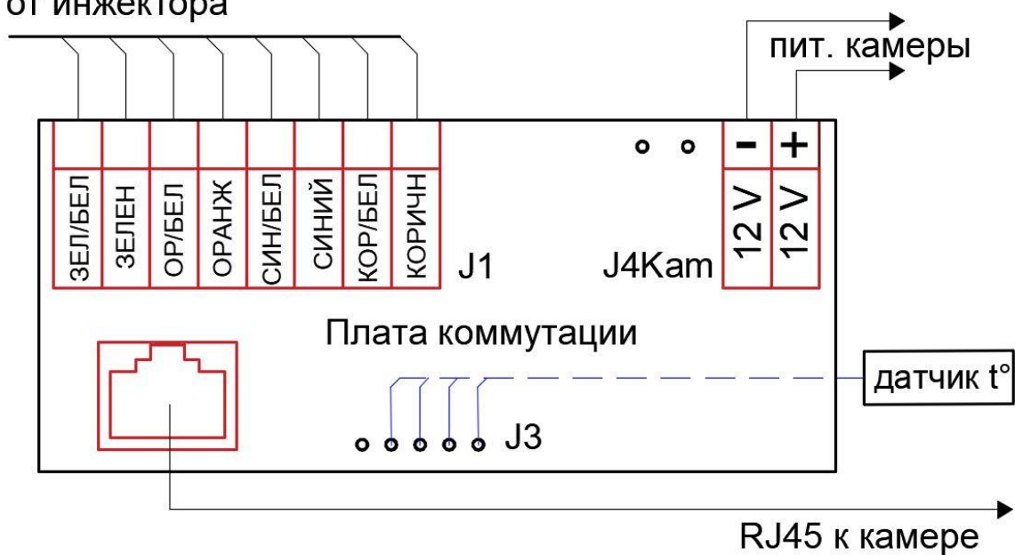
Рисунок 6в – Подключение термокожуха с питанием по PoE
