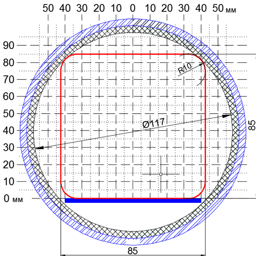
Рисунок 3 – Сечение термокожуха с ИК-прожектором
