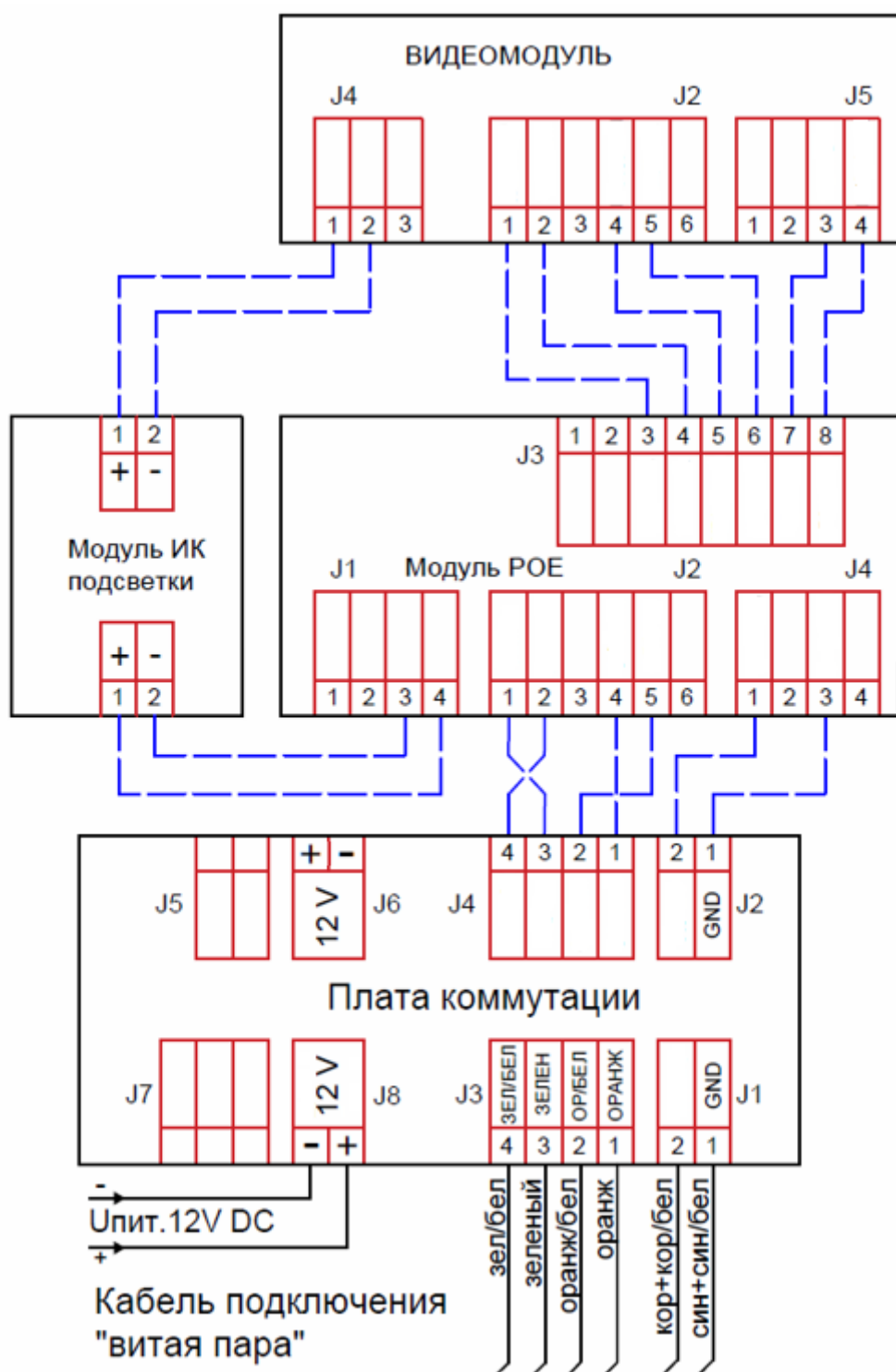
Рисунок 4 – Схема подключения камеры с питанием по PoE или 12В. По умолчанию видеокамера подключается с питанием по PoE на разъемы J1 и J3 «Платы коммутации» - без включения обогрева. При необходимости подключения обогрева подать напряжение 12V DC на клеммы разъема J8 «Платы коммутации», к клемме J6 «Платы коммутации» подключить подписанные заизолированные провода (красный – «+» и черный – «-»), идущие от платы «Модуль PoE».
