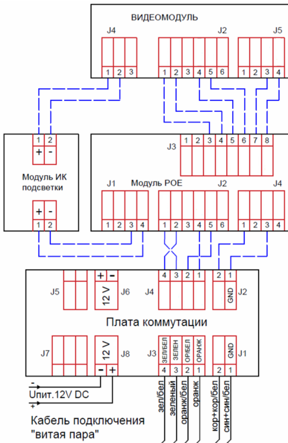
Рисунок 4 – Схема подключения камеры с питанием по PoE или 12V. По умолчанию видеочасть подключается с питанием по PoE на разъемы J1 и J3 «Платы коммутации» - без включения обогрева. При необходимости подключения обогрева подать напряжение 12V DC на клеммы разъема J8 «Платы коммутации», к клемме J6 «Платы коммутации» подключить подписанные изолированные провода (красный – «+» и черный – «-»), идущие от платы «Модуль PoE».
