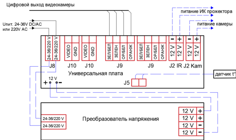
Рисунок 2 – Схема внешних подключения видеокамеры. Синей пунктирной линией указаны внутренние цепи.
