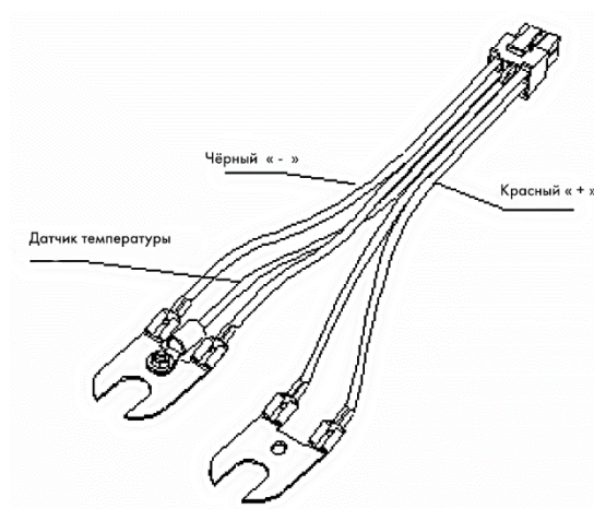
Рис. 2 Внешний вид кабеля
