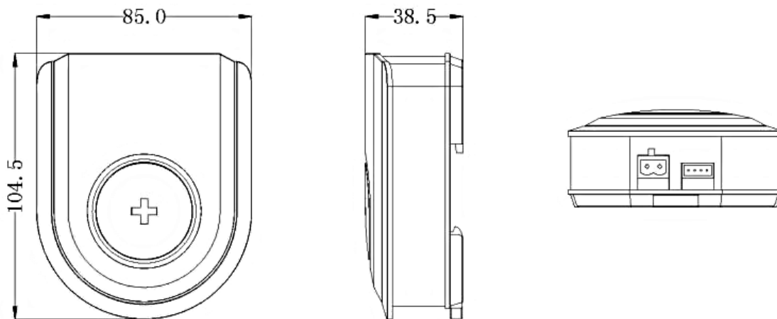
Рис.1 Внешний вид и габаритные размеры датчика
