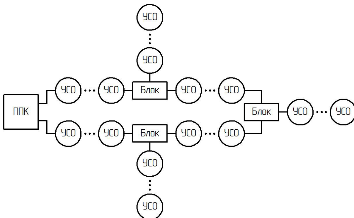
Рисунок 5 – Топология «Смешанная»
