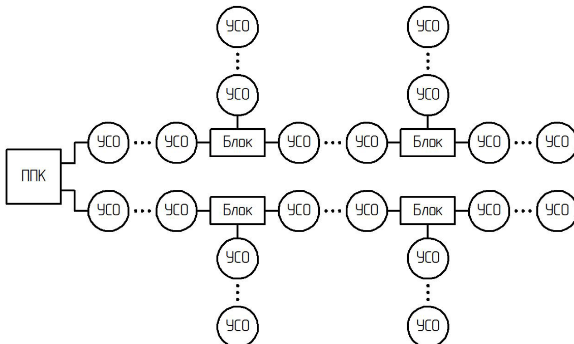
Рисунок 4 – Топология «Дерево»
