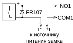
Рисунок 3 Схема подключения контроллера
