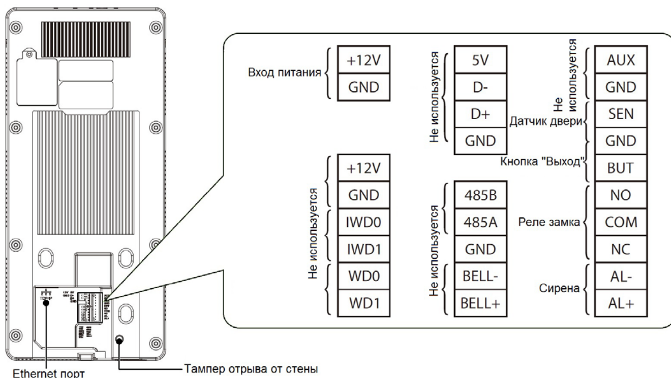
Рисунок 5. Схемы расположения разъёмов
