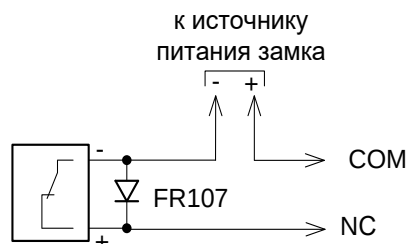
Рисунок 4. Схемы подключения контроллера
