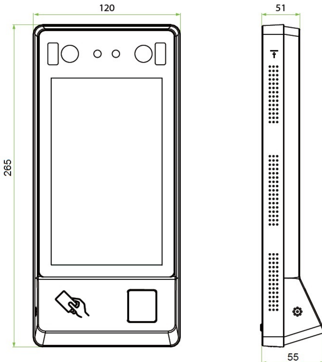
Рисунок 1. Внешний вид и габаритные размеры контроллера
