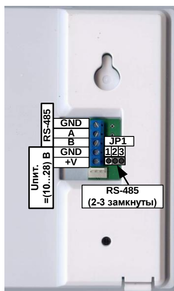
Рис. 3 Подключение (вид сзади).
