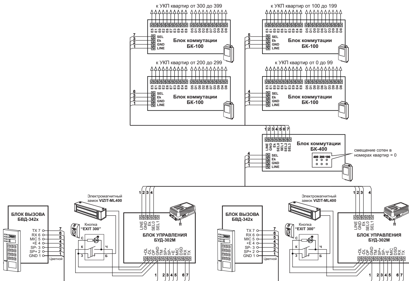
Рисунок 2 - Схема соединений блока коммутации БК-400
