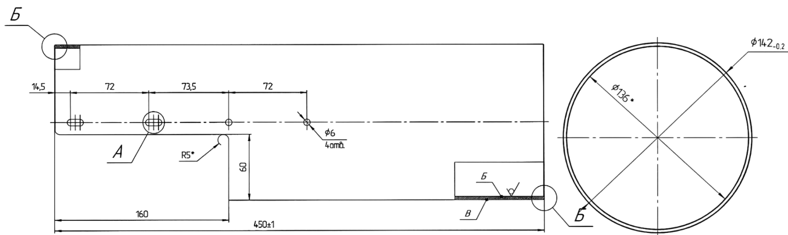
Рисунок А3. Габаритные размеры оптической бленды Спектрон-03-М для извещателей пламени «Спектрон-901-Exd-М/Н», «Спектрон-804-Exd-М/Н» и «Спектрон-801-Exd-М/Н» всех модификаций.
