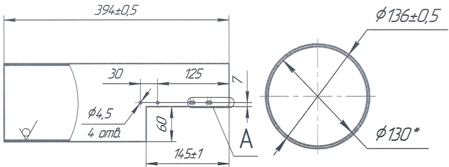
Рисунок А2. Габаритные размеры оптической бленды Спектрон-02-М для извещателей пламени «Спектрон-901-Exd-А», «Спектрон-804-Exd-А», «Спектрон-801-Exd-А», «Спектрон-601-Exd-А» и «Спектрон-401-Exd-А» всех модификаций.
