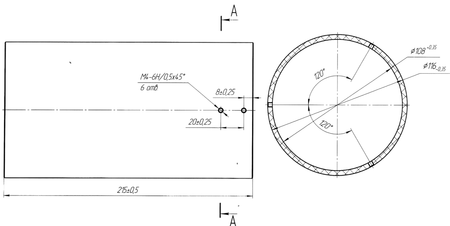
Рисунок А1. Габаритные размеры оптической бленды Спектрон-01-М для извещателей пламени «Спектрон-601-Exd-М/Н» и «Спектрон-401-Exd-М/Н» всех модификаций.
