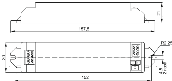
Рисунок 1 – БАП40-1,0
