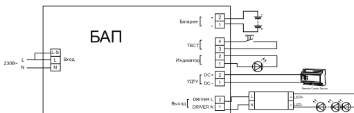
а) БАУ40-1,0
