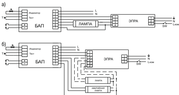
а) Схема подключения с ЭПРА для однолампового светильника
