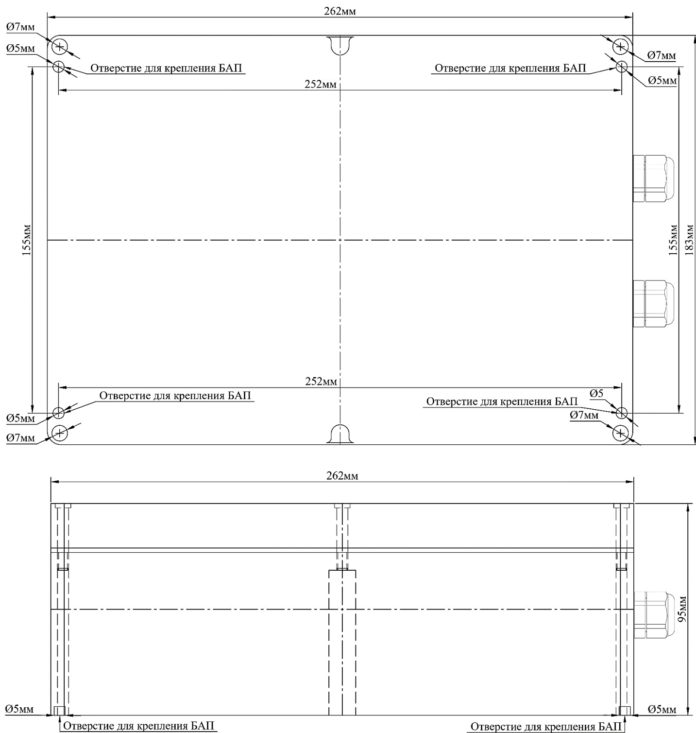
Рисунок 1-Габариты блока аварийного питания
