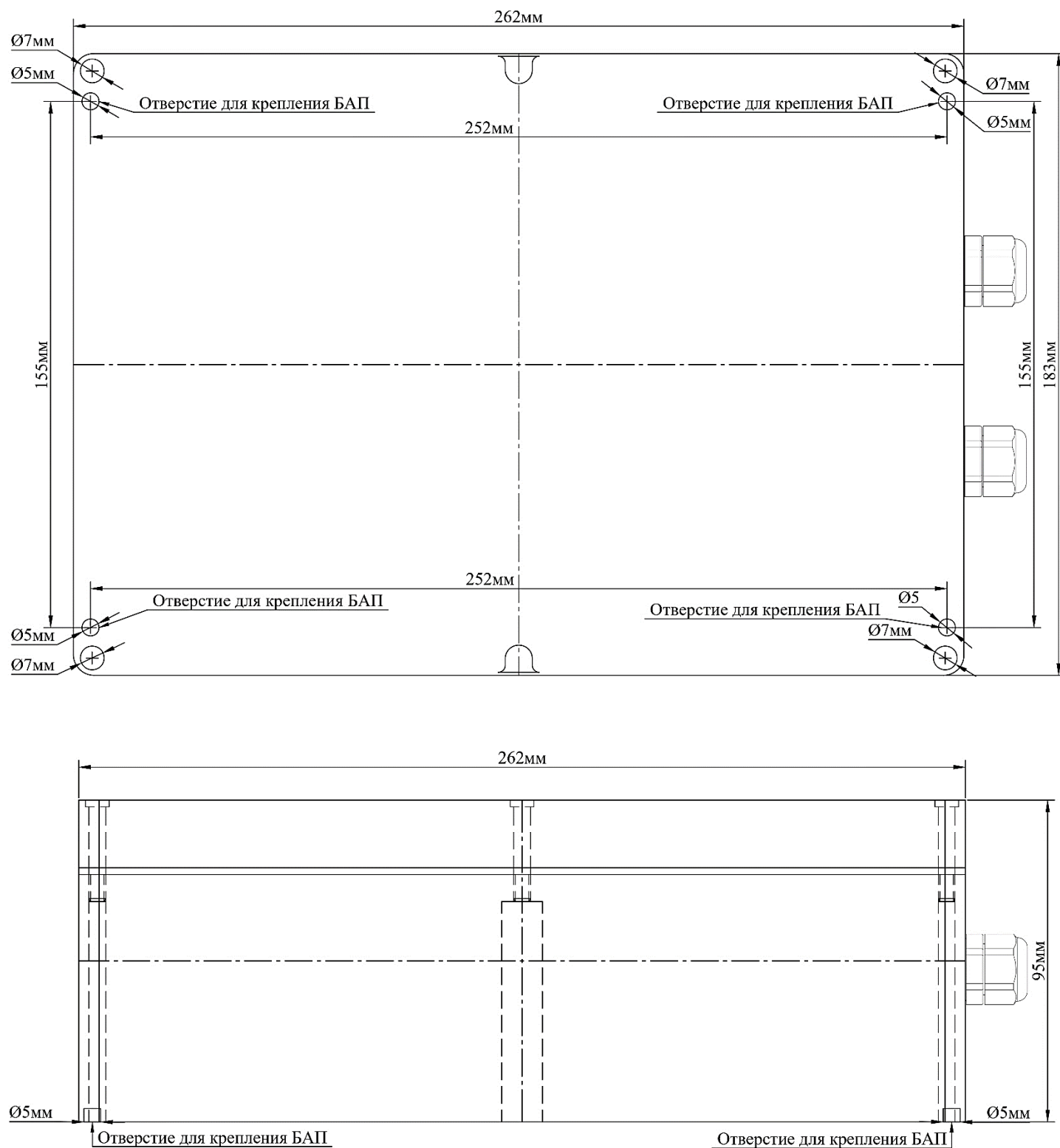
Рисунок 1-Габариты блока аварийного питания
