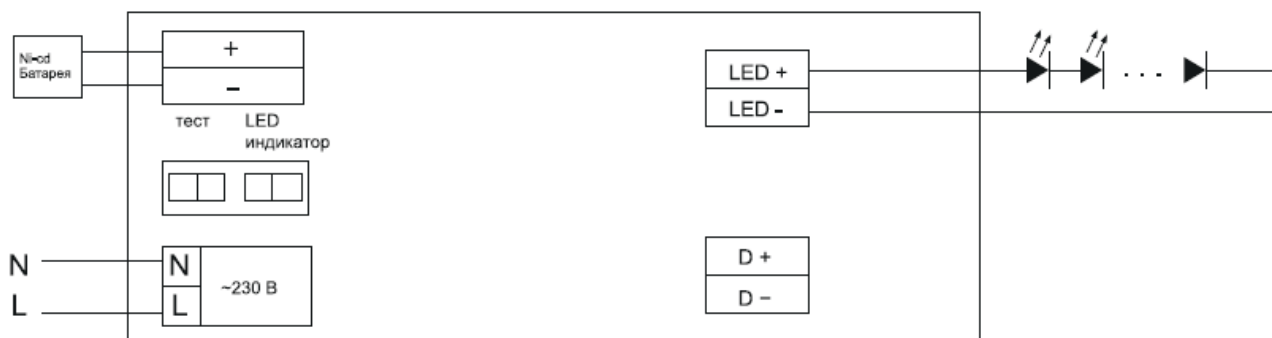
Рисунок 3 Подключение БАП (непостоянный аварийный светильник)
