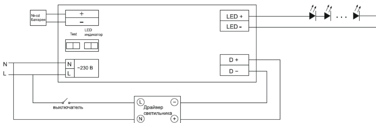
Рисунок 3 Подключение БАП (непостоянный аварийный светильник)
