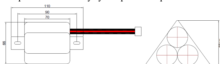
Габаритная схема аккумуляторной батареи
