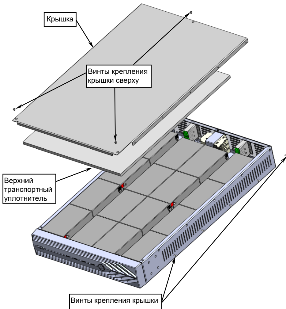
Рисунок 7 — Замена аккумуляторных батарей.
