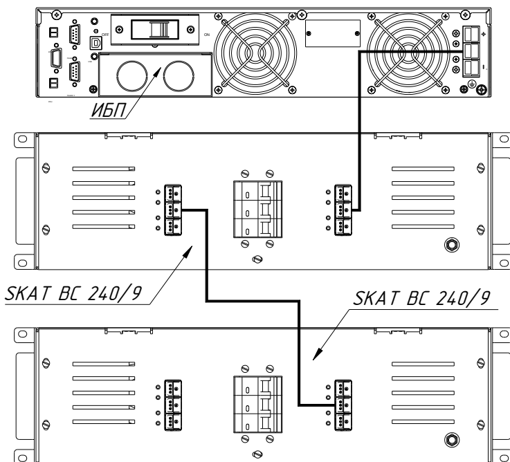
Рисунок 5 — Подключение ИБП и дополнительного батарейного блока
