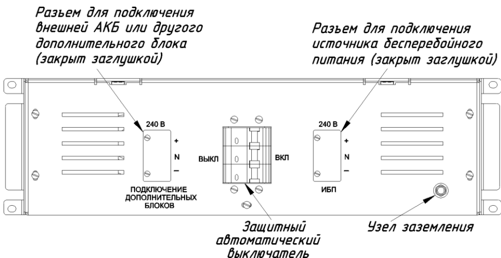
Рисунок 2 – Общий вид задней панели изделия
