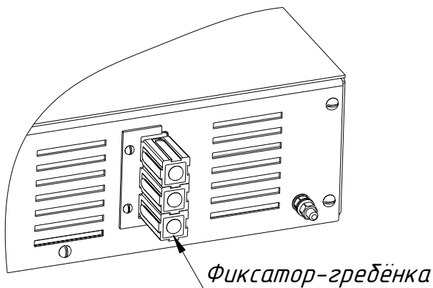
Рисунок 6 — Подключение кабельного разъема к изделию
