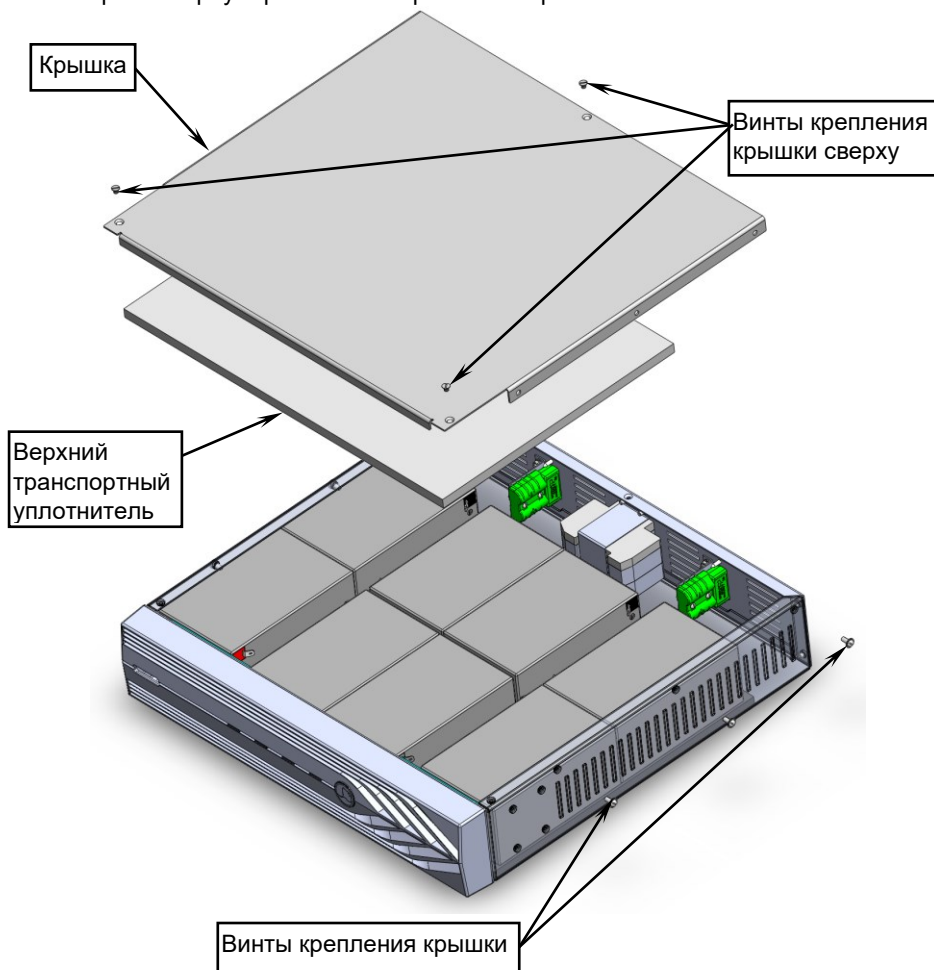
Рисунок 6 — Замена аккумуляторных батарей.
