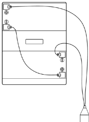
Рисунок 9 – Схема соединений АКБ в группе изделия SKAT BC 24/18S3 RACK P3
