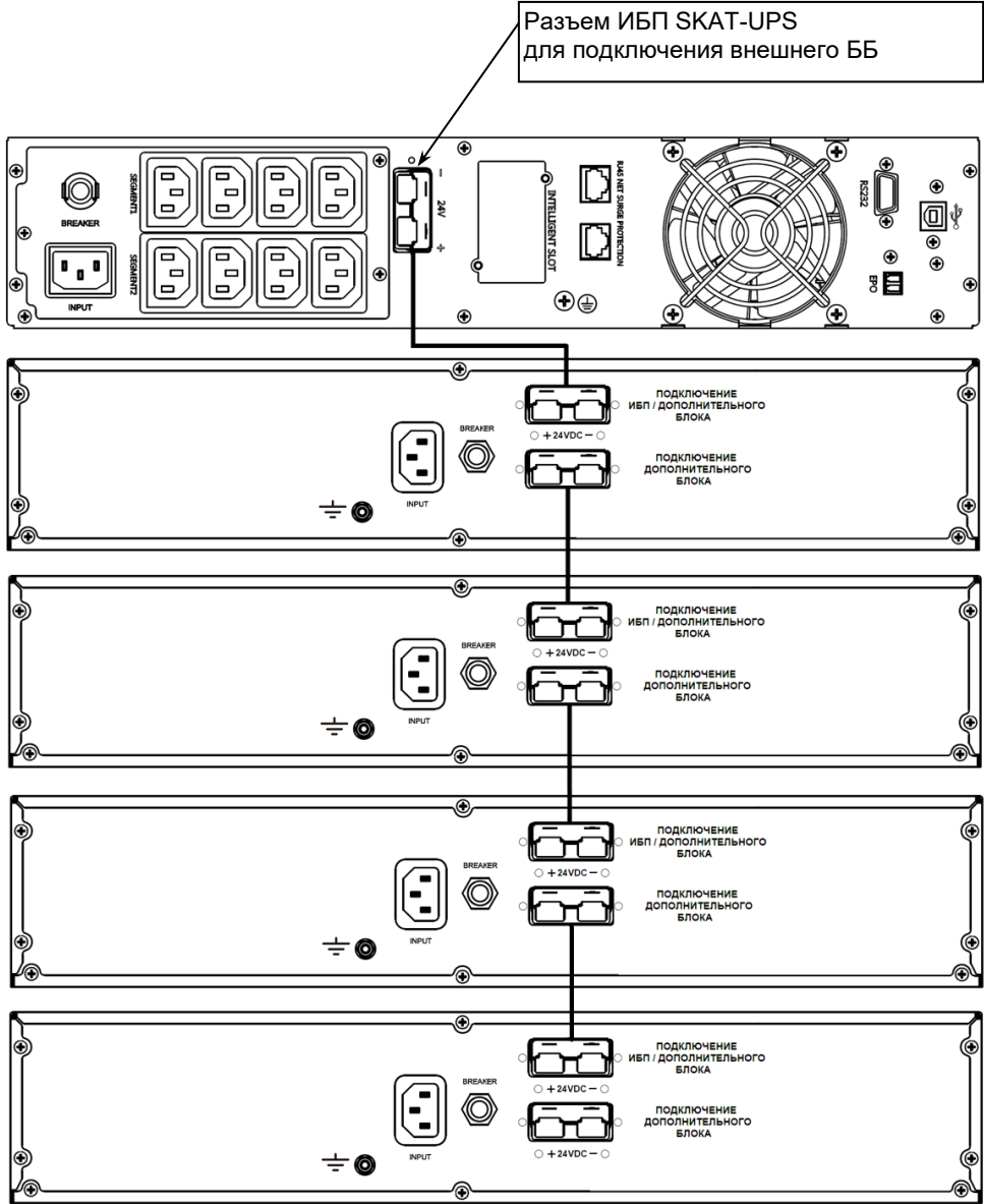
Рисунок 6 – Схема подключения нескольких ББ к ИБП (Продолжение на стр. 11)
