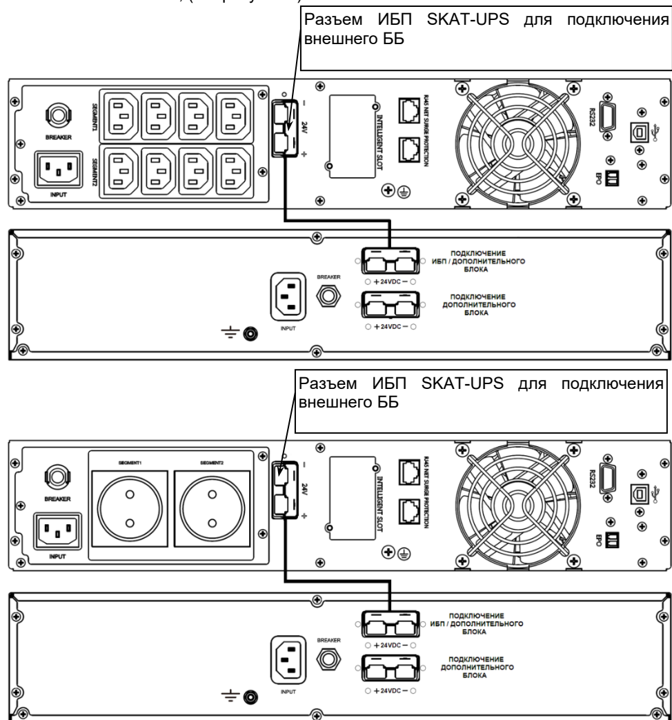
Рисунок 5 – Схемы подключения ББ к ИБП SKAT-UPS
