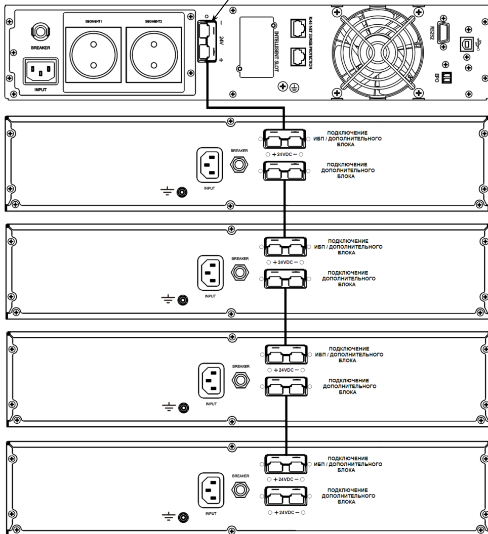
Рисунок 6 – Схема подключения нескольких ББ к ИБП (Начало на стр. 10)
