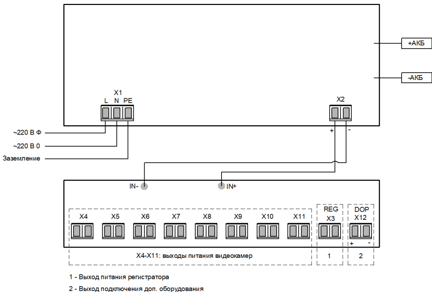
Рисунок 1 – схема подключения.
