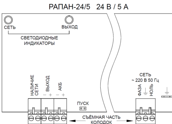
Рисунок 2 - Общий вид платы
