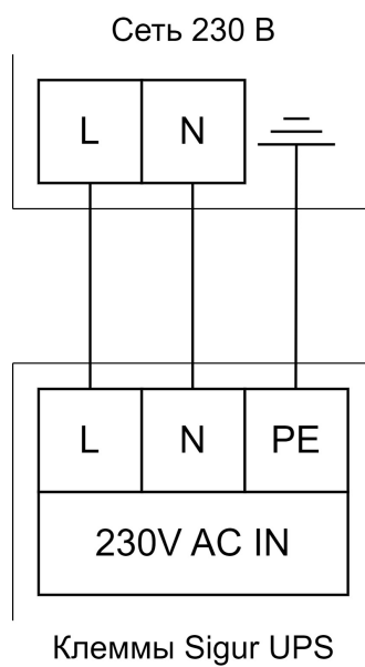
Схема подключения устройства к сети переменного напряжения.
