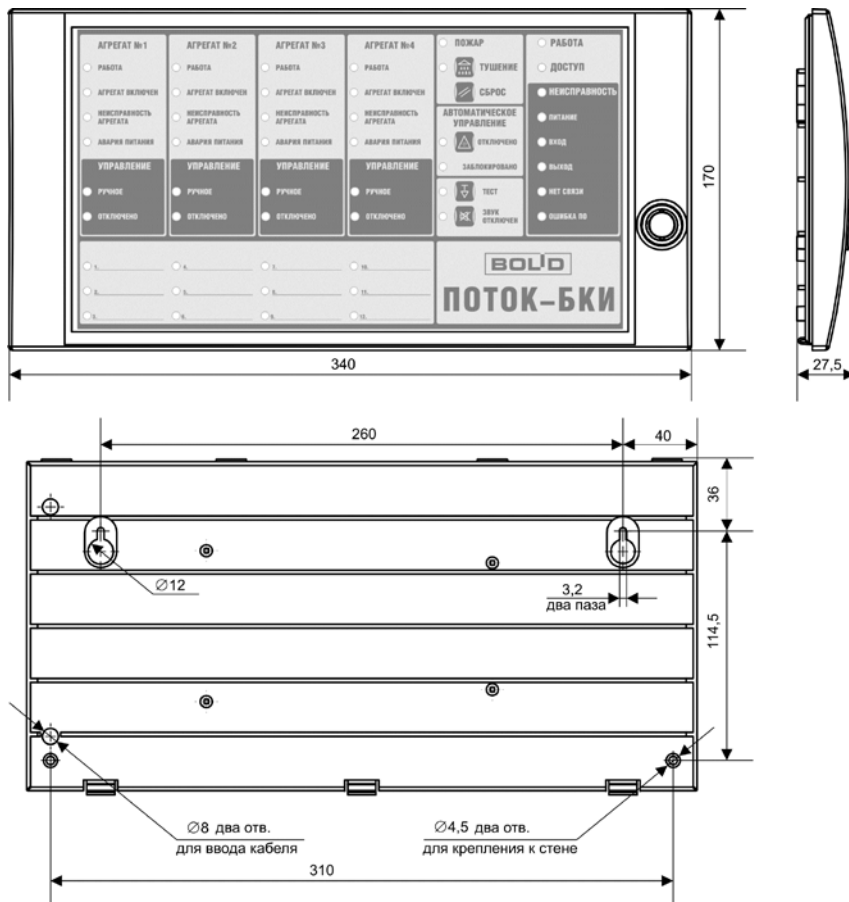
Рисунок 1. Внешний вид, габаритные и установочные размеры блока «Поток-БКИ»
