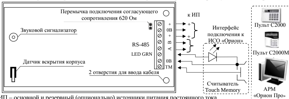
Рисунок 3. Схема внешних соединений блока
