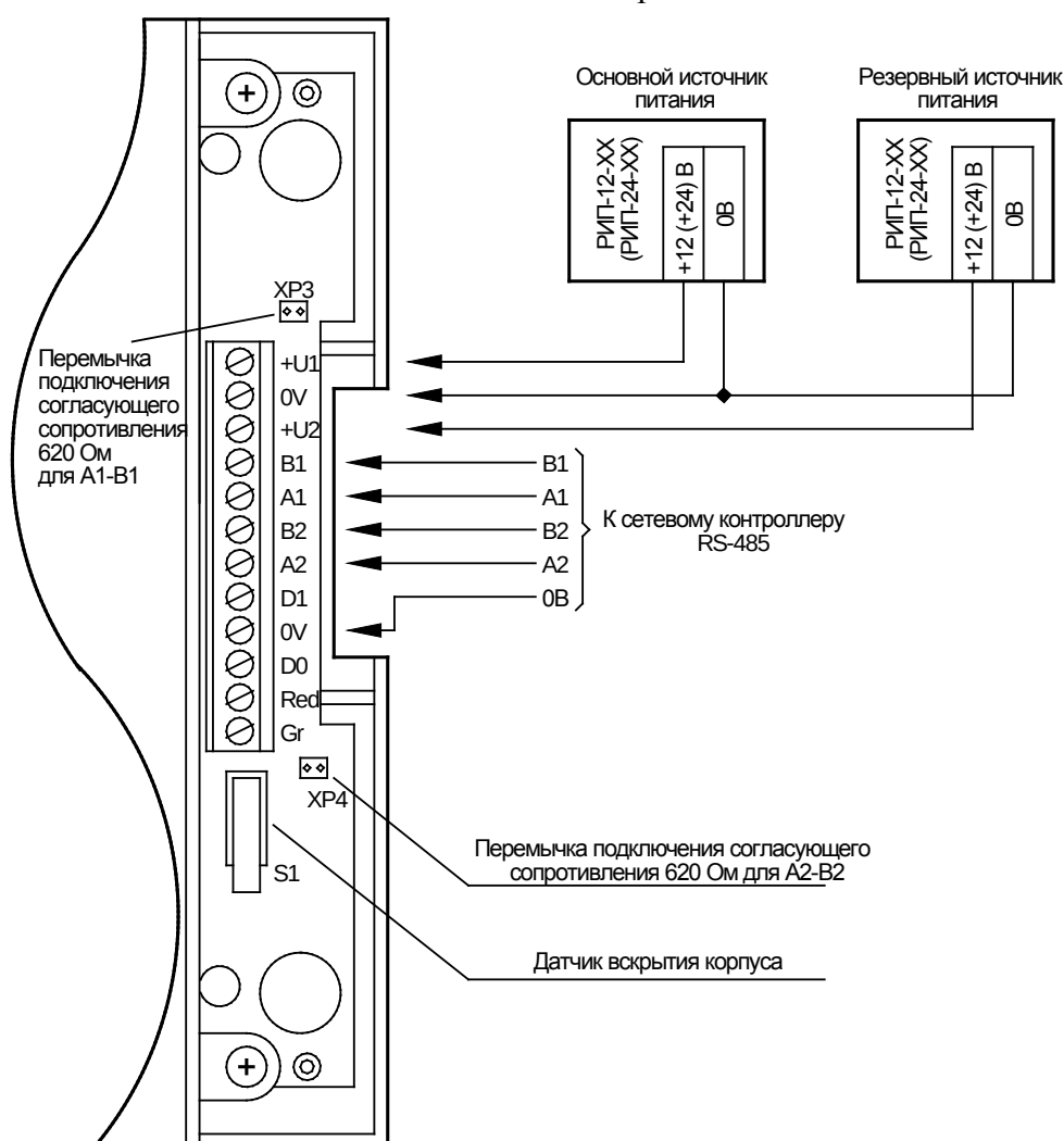
Рисунок 2. Схема внешних соединений блока «C2000-ПТ 2RS485»
