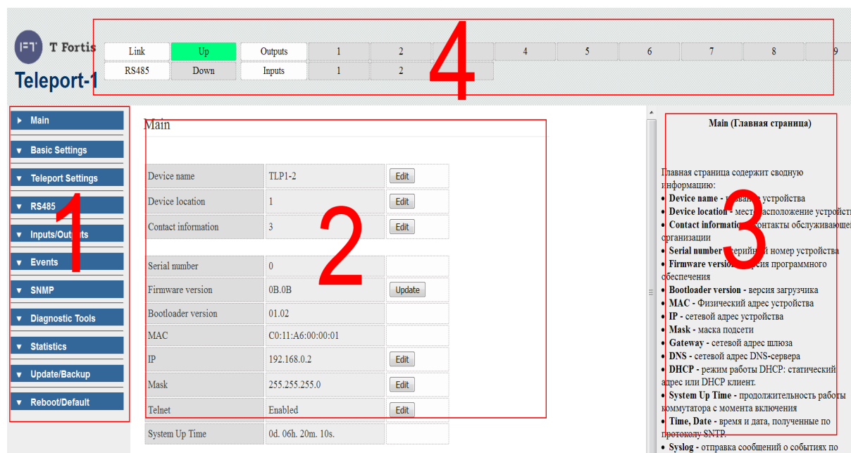
Рис. 5.3.1.2. Web-интерфейс
