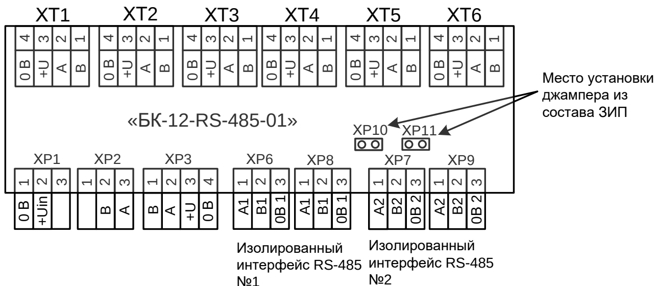
БК-12-RS-485-01 с открытой крышкой
