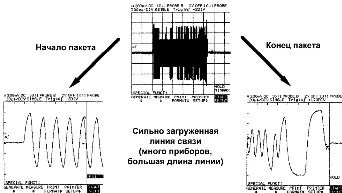
Рисунок 60 Типичная осциллограмма сигнала при большой загрузке линии связи
