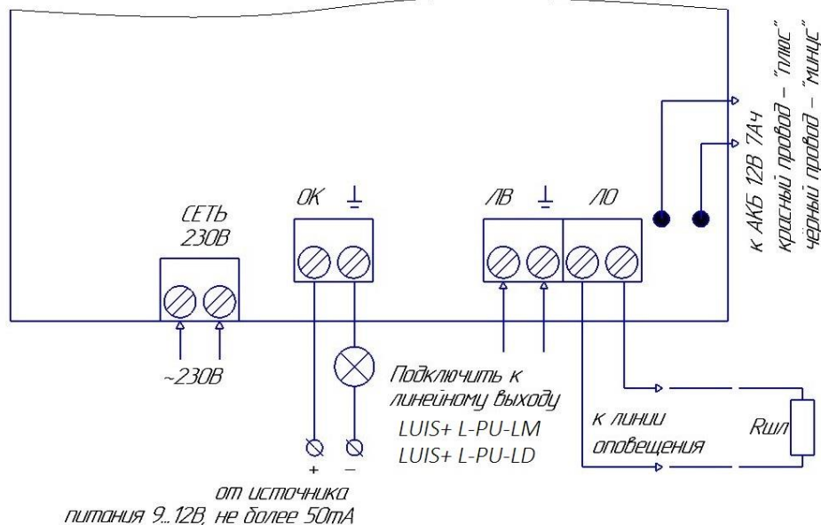
Рисунок 1. Схема внешних соединений прибора «LUIS+ L-PU-L»
