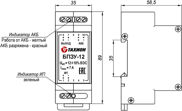
Рис.1 Габаритные размеры
