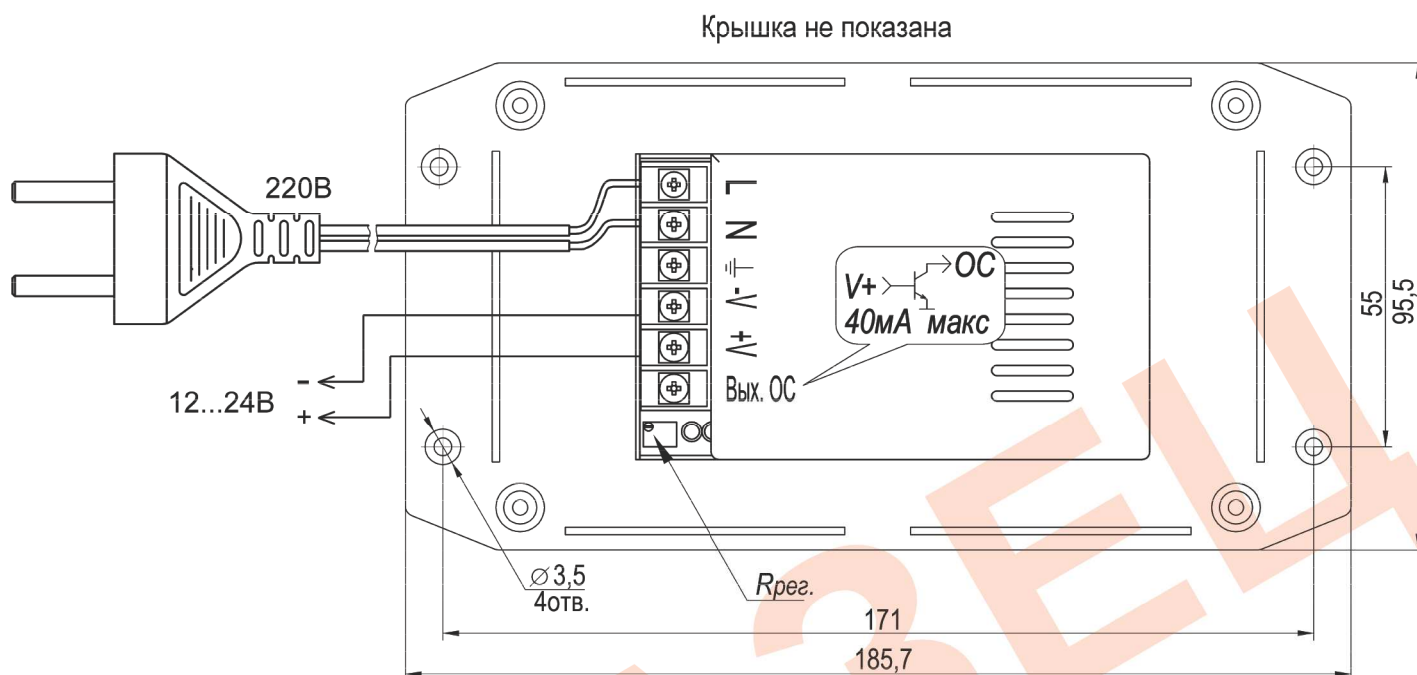
Рис.1 Устройство, габаритные и установочные размеры, подключение изделия
