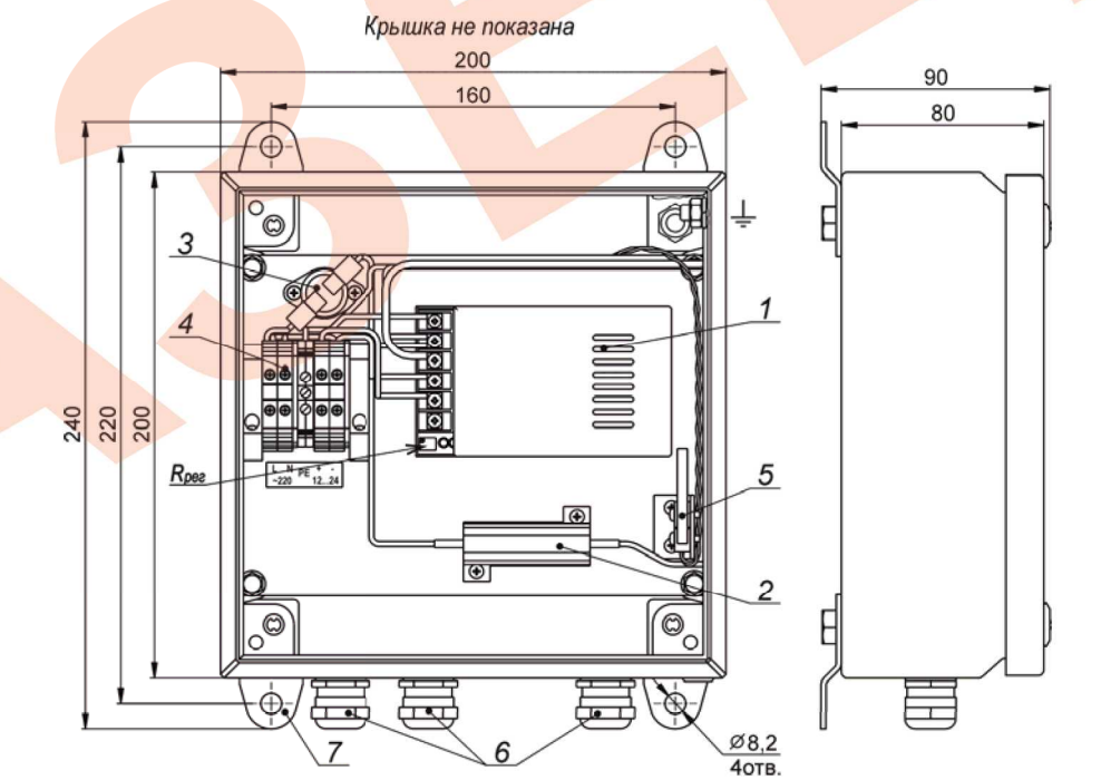
Рис.1 Устройство, габаритные и установочные размеры БПУ-1
