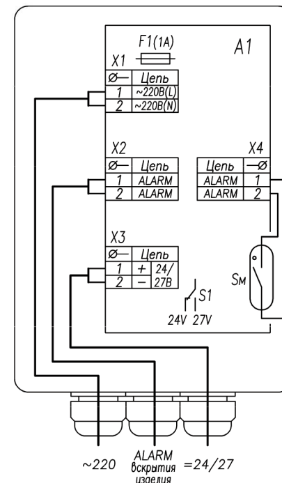
Рис.2 Схема электрическая принципиальная
