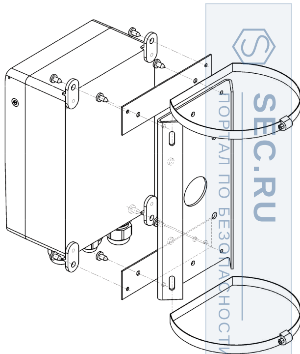
Рис.3 Монтаж кронштейна для крепления на опору
