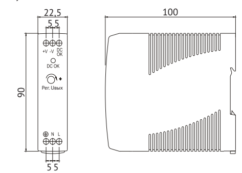
Рис.2 Габаритные размеры блоков питания MDR-10, 20
