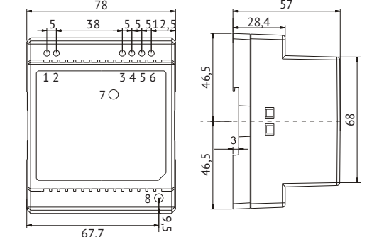
Рис.5 Габаритные размеры блоков питания DR-15
