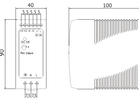
Рис.3 Габаритные размеры блоков питания MDR-40, 60
