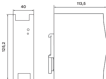
Рис. 3 Габаритные размеры блока питания, DR-E-120W-12/24
