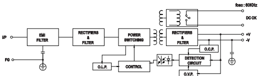
Рис 4. Блок схема DR-M-40W-5/12/24, DR-M-60W-5/12/24
