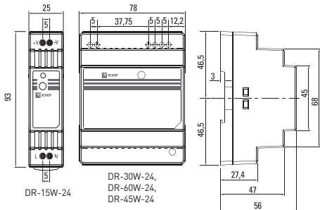
Рис. 3 Габаритные размеры блока питания.
