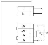
Рис. 1 Схема подключения блока питания мощностью 15-60 ватт.
