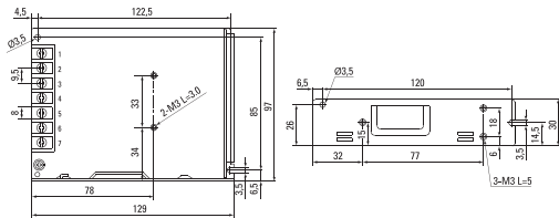
Рис 3. Габаритные размеры (MPS-100W-24)
