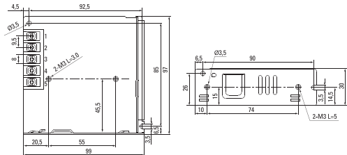
Рис 2. Габаритные размеры (MPS-75W-24)
