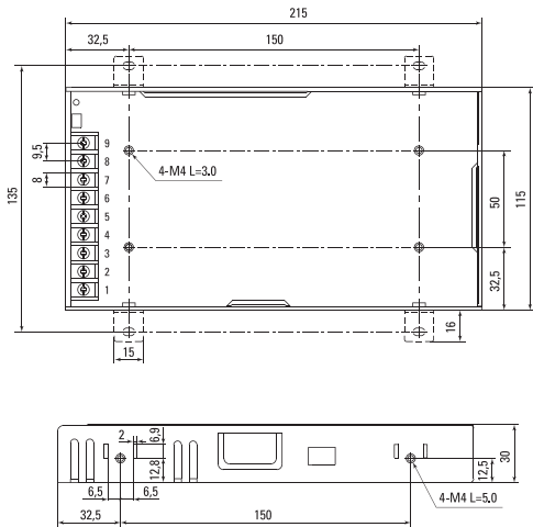
Рис 5. Габаритные размеры (MPS-200W-24, MPS-350W-24)
