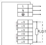
Рис 9. Схема подключения (MPS-200W-24, MPS-350W-24, MPS-500W-24)
