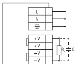
Рис 8. Схема подключения (MPS-100W-24, MPS-150W-24)
