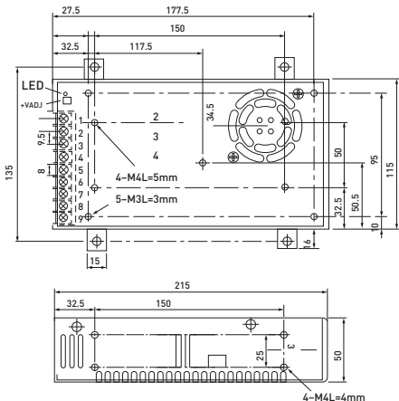
Рис 6. Габаритные размеры (MPS-500W-24)
